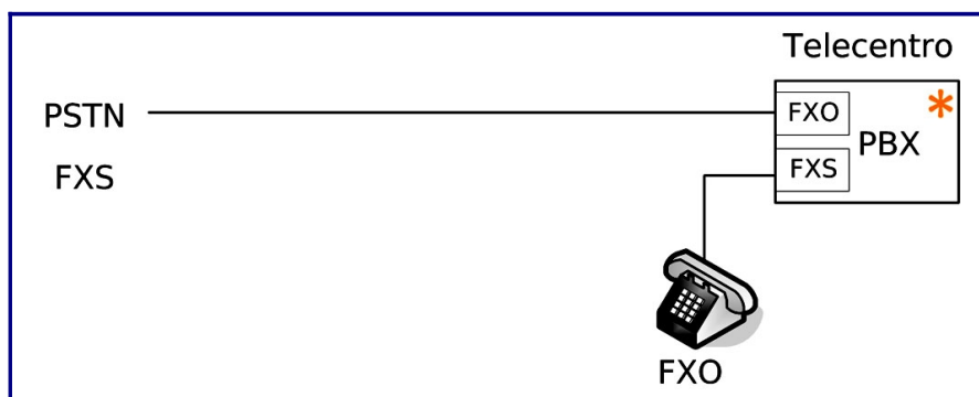
Figura 9: El Telecentro usa una tarjeta TDM400P wildcard para (1) conectar la PBX a la RTB (módulo FXO) y (2) añadir una extensión al teléfono analógico (FXS module).
