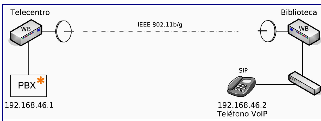
Figura 5: La biblioteca comunitaria está conectada a la PBX a través de una pasarela inalámbrica.
