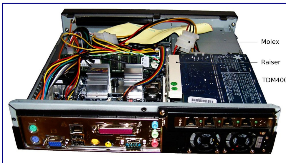
Figura 4: Una central telefónica portátil basada en una placa mini-ITX con una tarjeta Digium TDM400P
