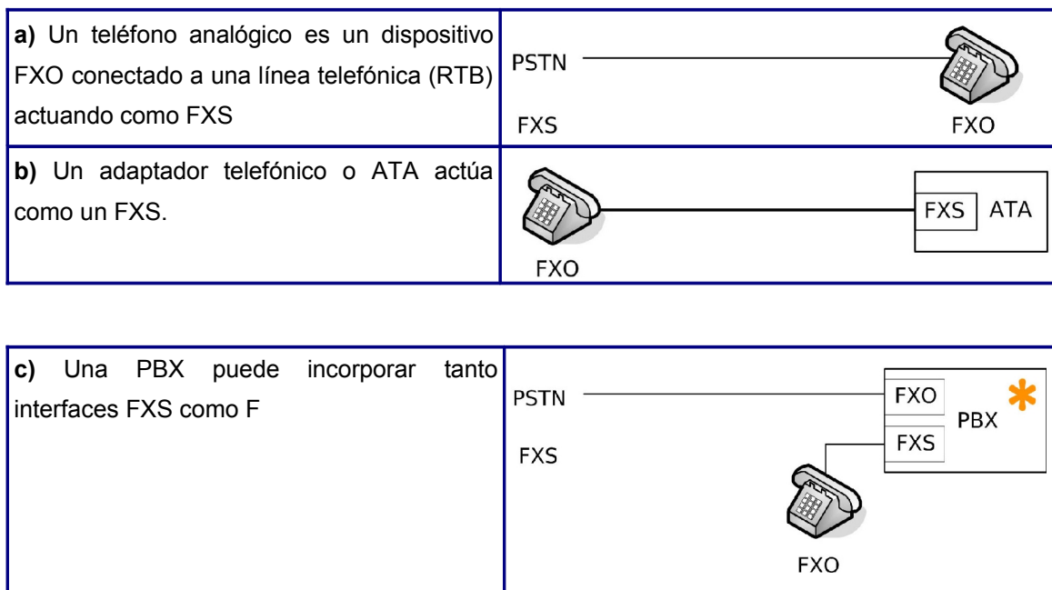
Figura 1: Telefonía tradicional a),b) y c)
