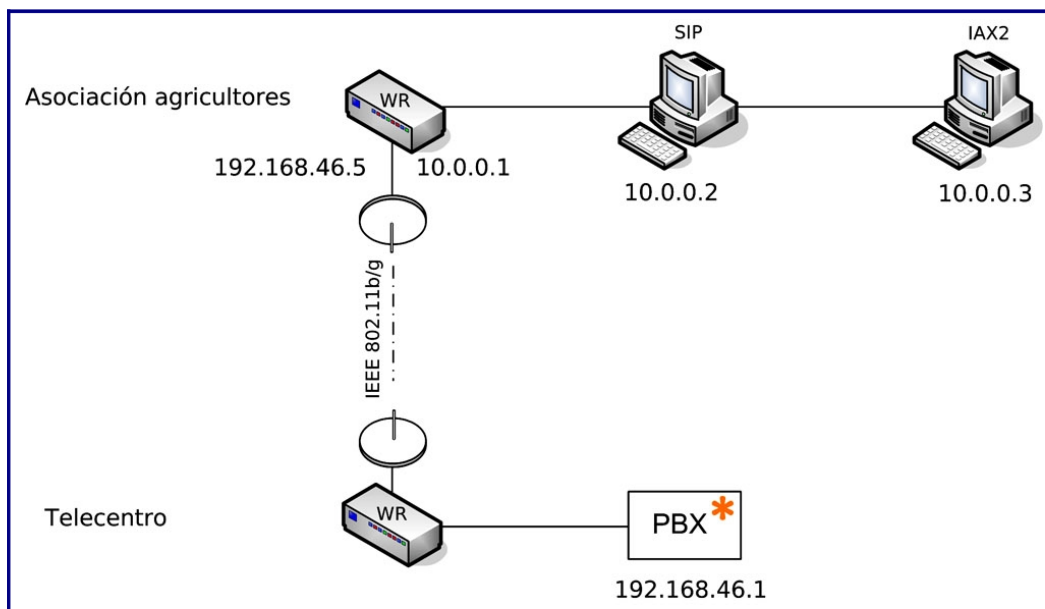
Figura 8: La asociación de agricultores está conectada a la centralita a través de un NAT inalámbrico. Un programa de telefonía “soft phone” está instalado en cada uno de los computadores. El primer cliente usa el protocolo SIP mientras que el segundo usa IAX2.
