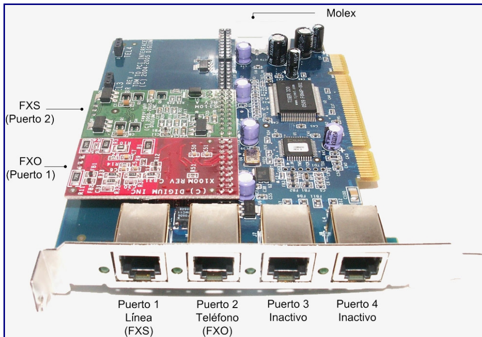
Figura 3: Una tarjeta TDM400P con sus cuatro puertos. Los dos primeros puertos (Puerto 1: FXO, Puerto 2: FXS) están ocupados mientras que los dos últimos puertos (Puerto 3 y 4) están inactivos.
