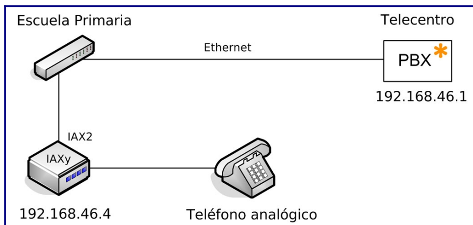
Figura 7: La escuela primaria está conectada a la PBX a través de un cable de par trenzado.
