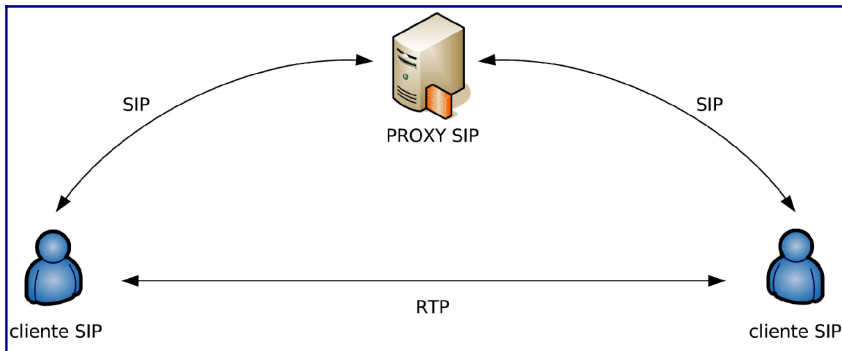
Figura 2: El proceso de registro entre clientes y el servidor “proxy”. La señalización (SIP) y las conversaciones de voz (RTP) viajan por caminos diferentes.
