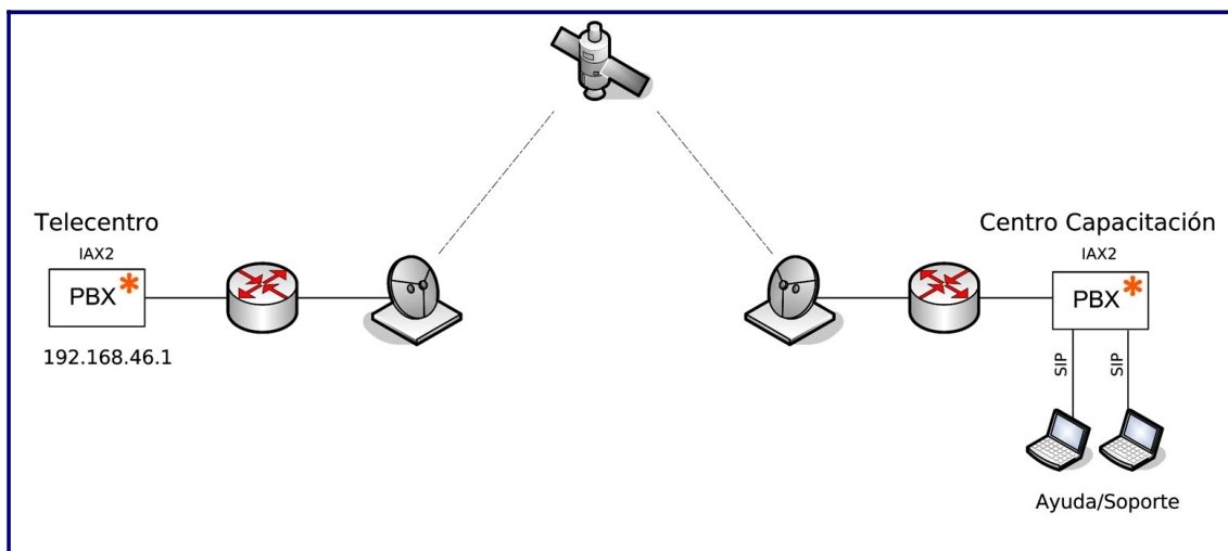
Figura 10: Tanto el Telecentro como el Centro de Capacitación tienen su centralita Asterisk . Las centralitas están interconectadas gracias a un enlace de satélite tipo VSAT.
